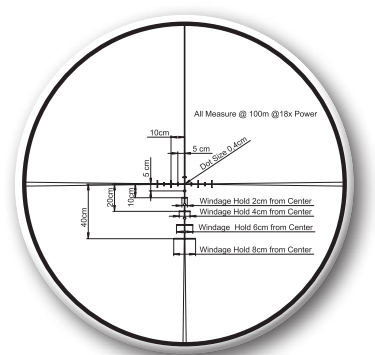
Прицел S3-I
