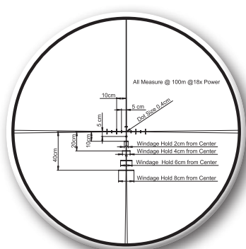
Absehen S3-I
